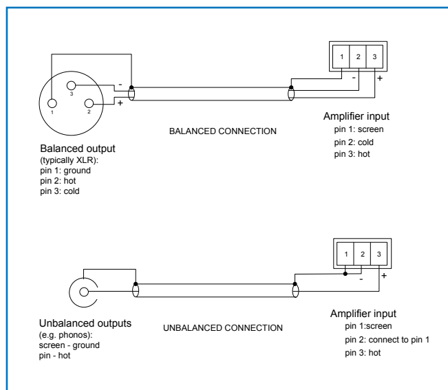
fig.4: Input Wiring
